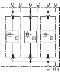
Schéma vnitřního zapojení DV M TNC 255
