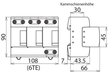
Rozměry DV M TNC 255
